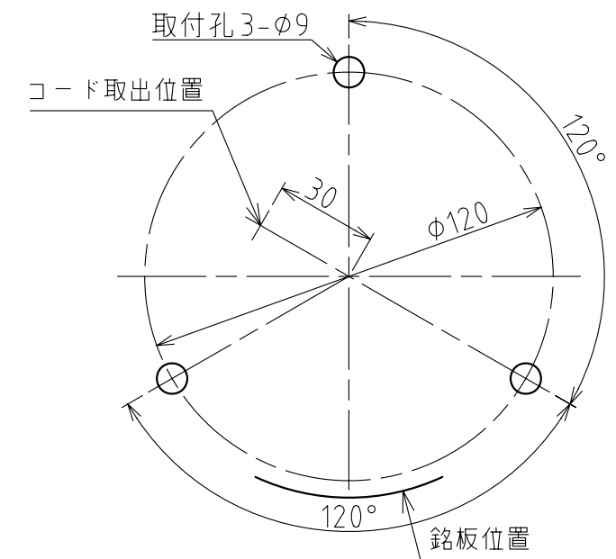
取付面寸法図 (尺度 1:2)
