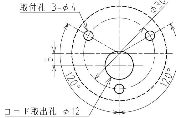
取付面寸法図 (1/1)
