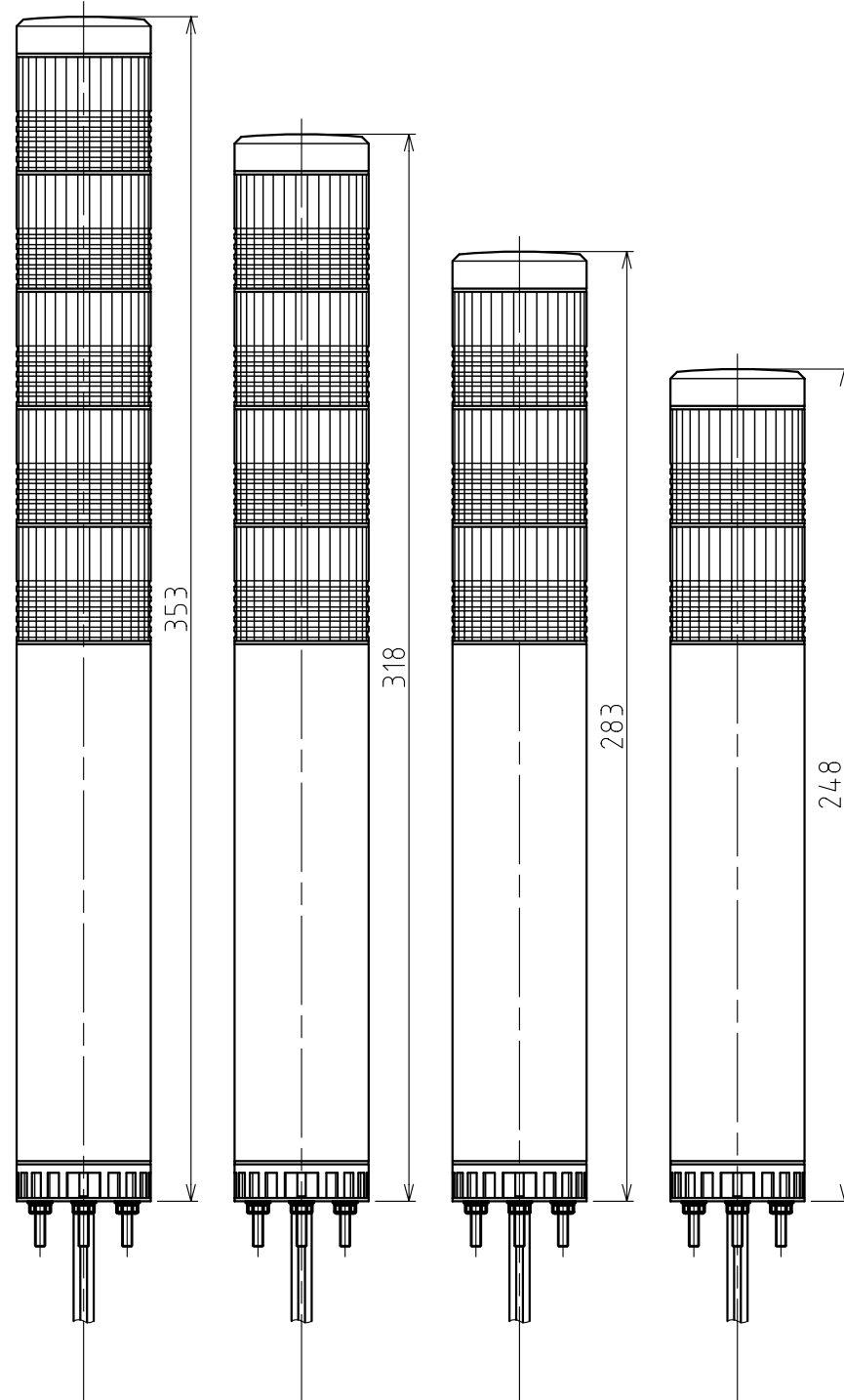
外観寸法図
