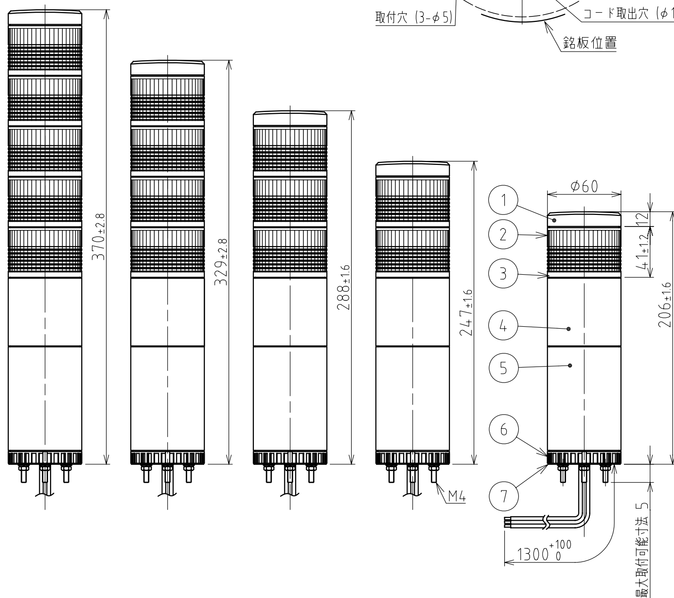
外観寸法図
