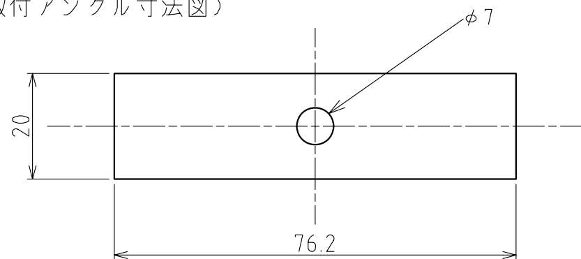
(取付アングル寸法図)
