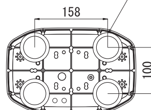
底面図 (マグネット式)
