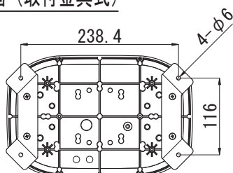
底面図 (取付金具式)
