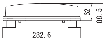
側面図 (取付金具式)
